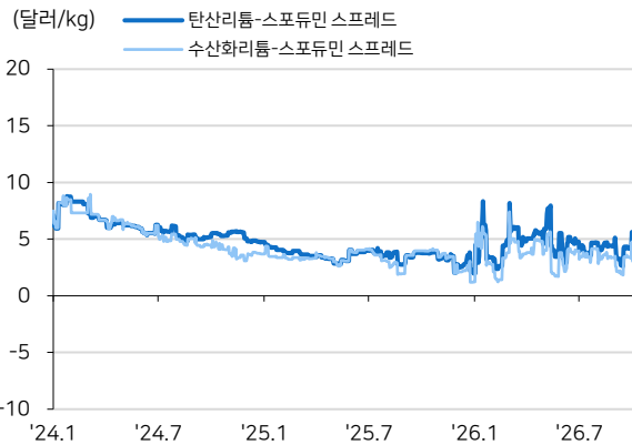
그림3 리튬-스포듀민 스프레드
