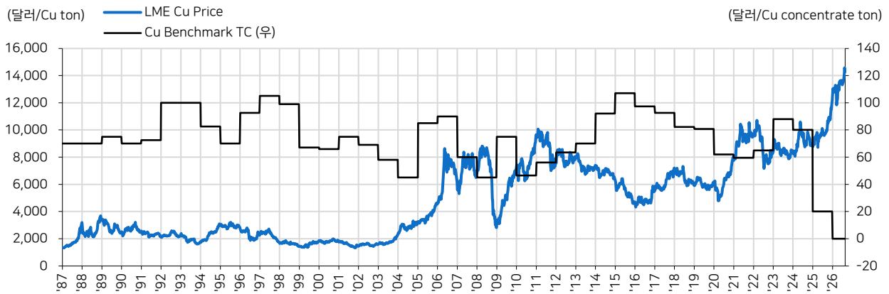
그림5 1987~현재까지의 구리 가격 및 Benchmark TC 추이
